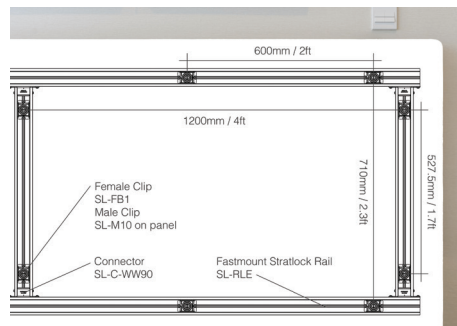
Solución de montaje de paneles: SL-FB1, SL-RLE y SL-C-WW90 - estructura y SL-M10 - panel
