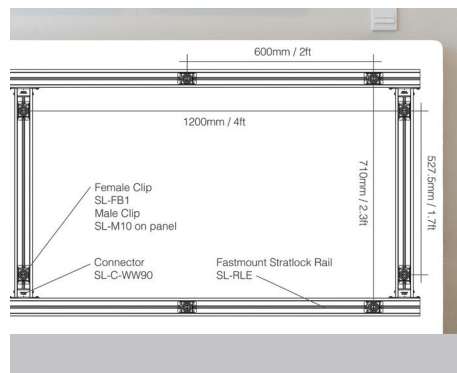
Solução de montagem de painéis: SL-FB1, SL-RLE e SL-C-WW90 - estrutura e SL-M10 - painel
